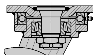
LSD sorozat - hegesztett acél nagy teherbírású iker-forgóvillák, megerősített forgófejű kivitel
