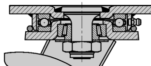
LS sorozat - hegesztett acél nagy teherbírású forgóvillák, megerősített forgófejű kivitel
