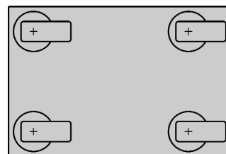
Négy forgóvillás kerék, azonos beépítési magasságban
