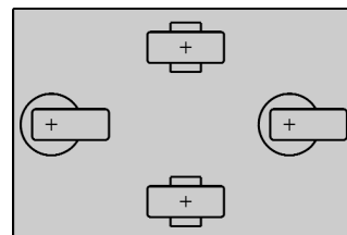
Két forgóvillás, két fixvillás görgő, ahol a fixvillás görgők beépítési magassága kicsit nagyobb
