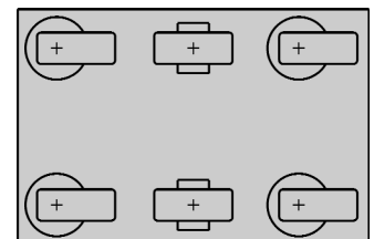
Négy forgóvillás és két fixvillás görgő azonos beépítési magasságban
